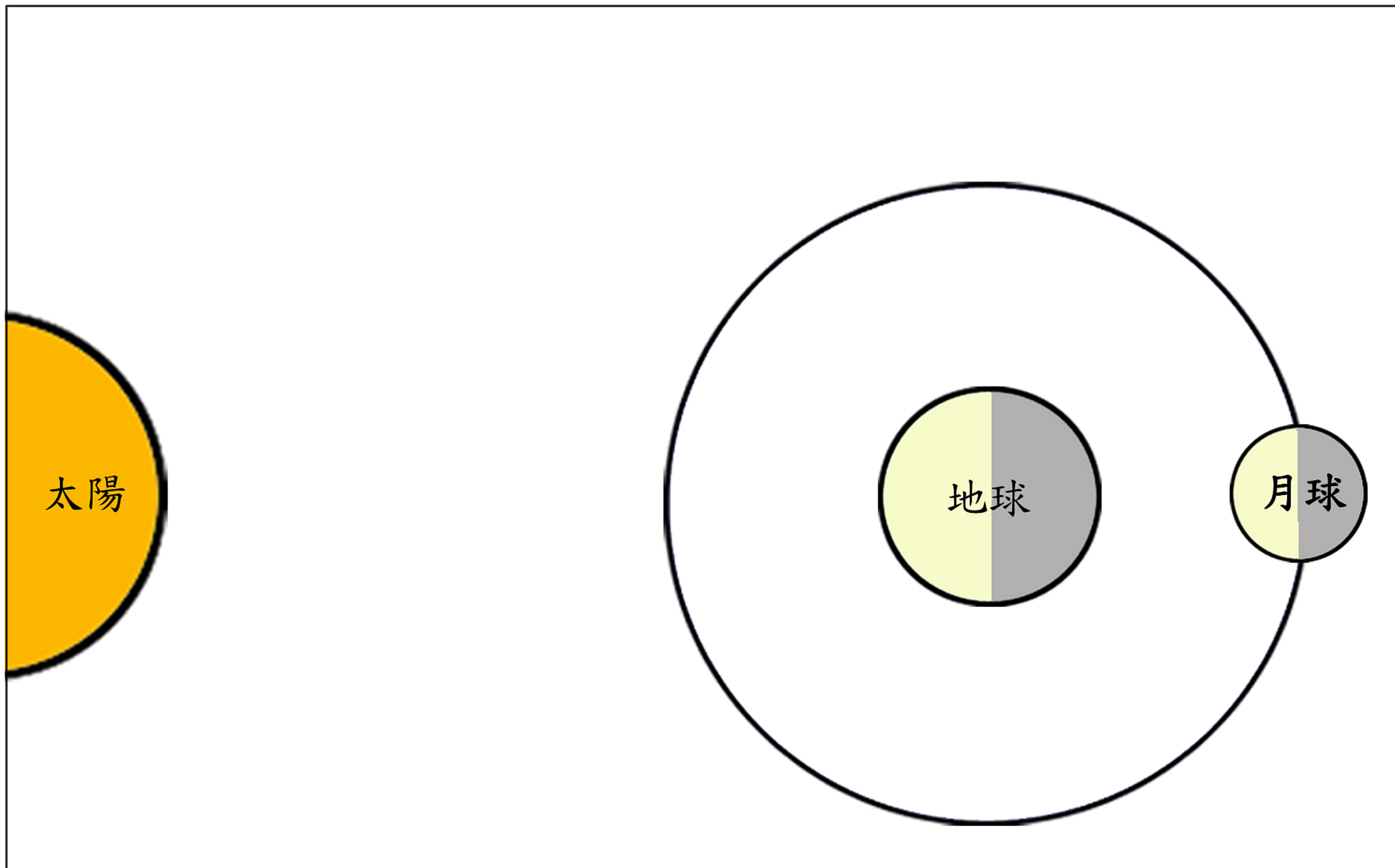
望月時太陽、地球及月球的位置
