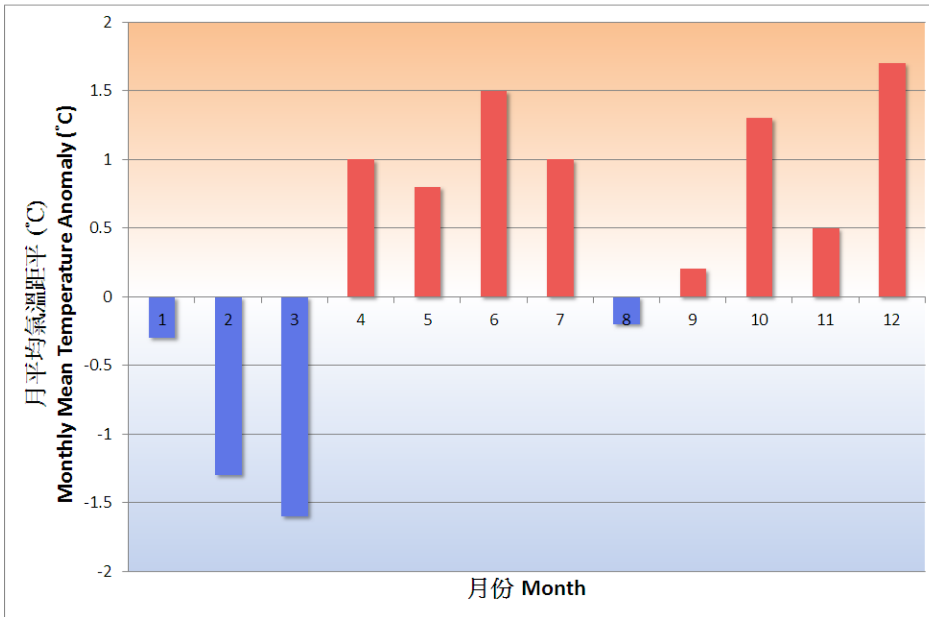
圖表一 二〇一六年香港月平均氣溫距平
