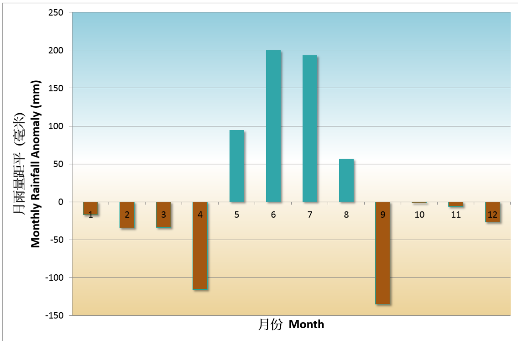
圖表五 二〇一七年香港月雨量距平
