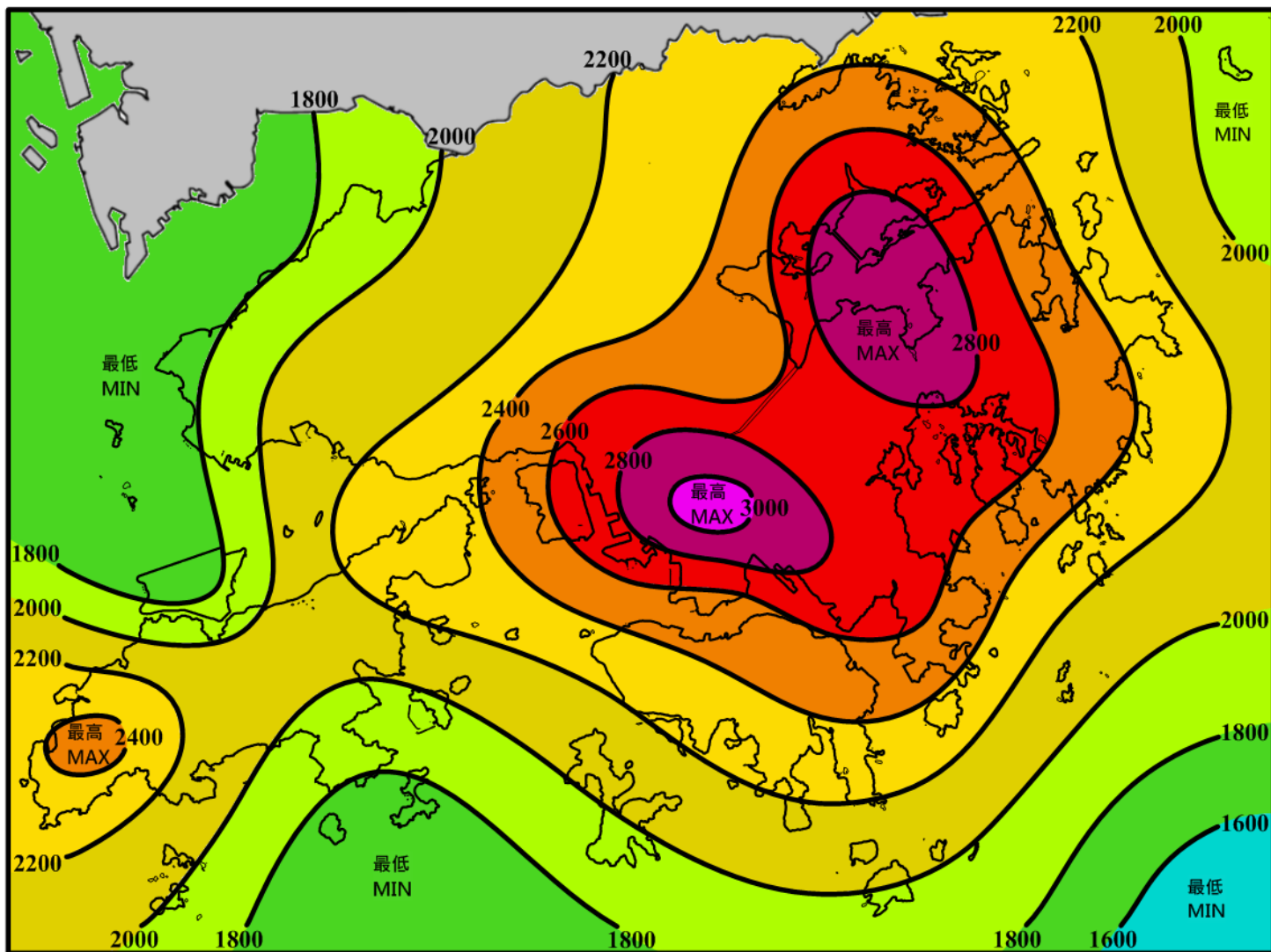
圖表六 二〇一七年香港年雨量(毫米)分布
