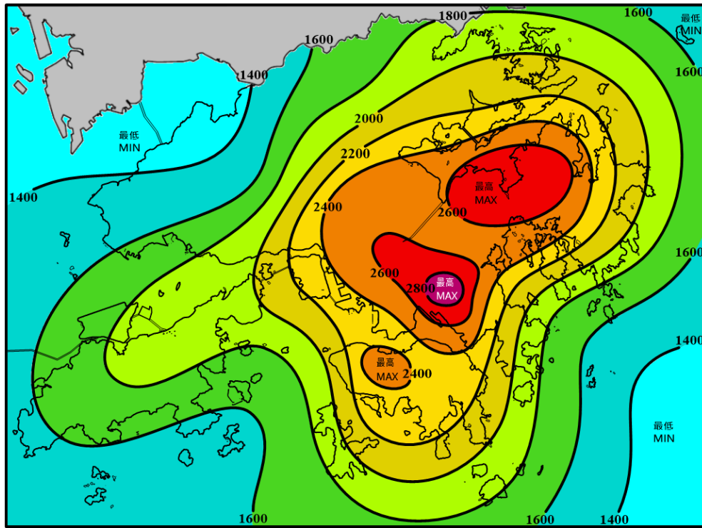
圖表七 二〇二〇年香港年雨量(毫米)分布
