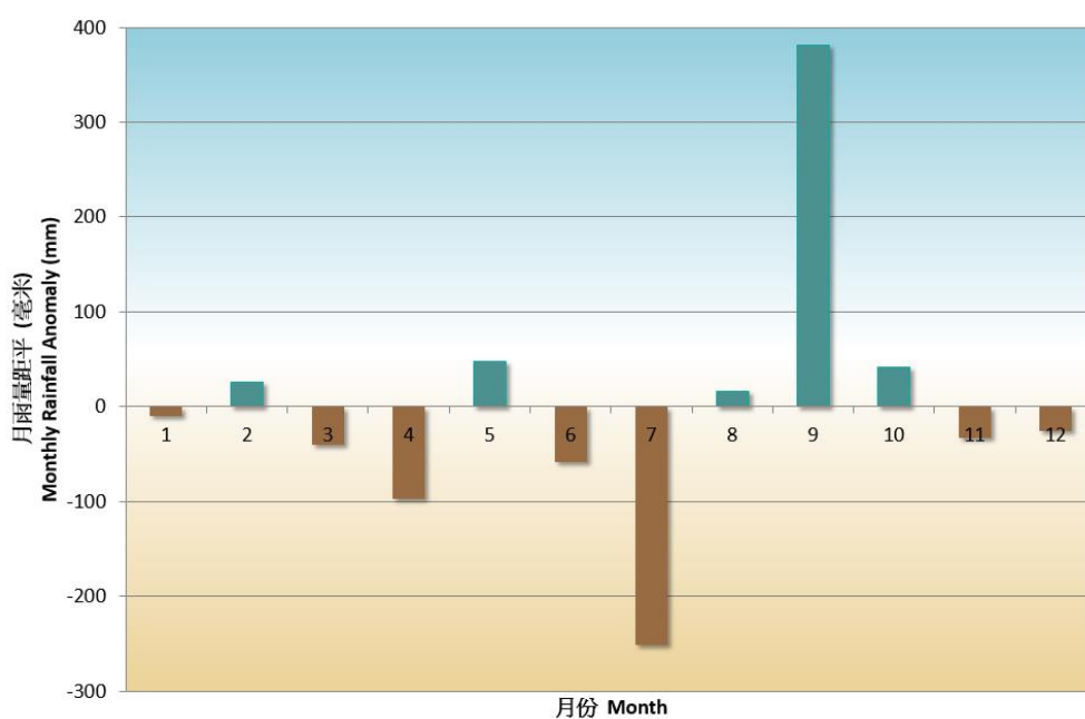
圖表六 二〇二〇年香港月雨量距平(與一九八一至二〇一〇年正常值相比)
