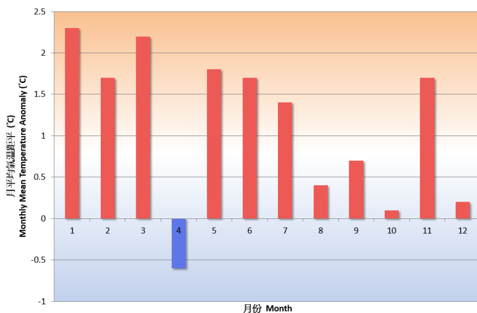
圖表一 二〇二〇年香港月平均氣溫距平與（與一九八一至二〇一〇年正常值相比）
