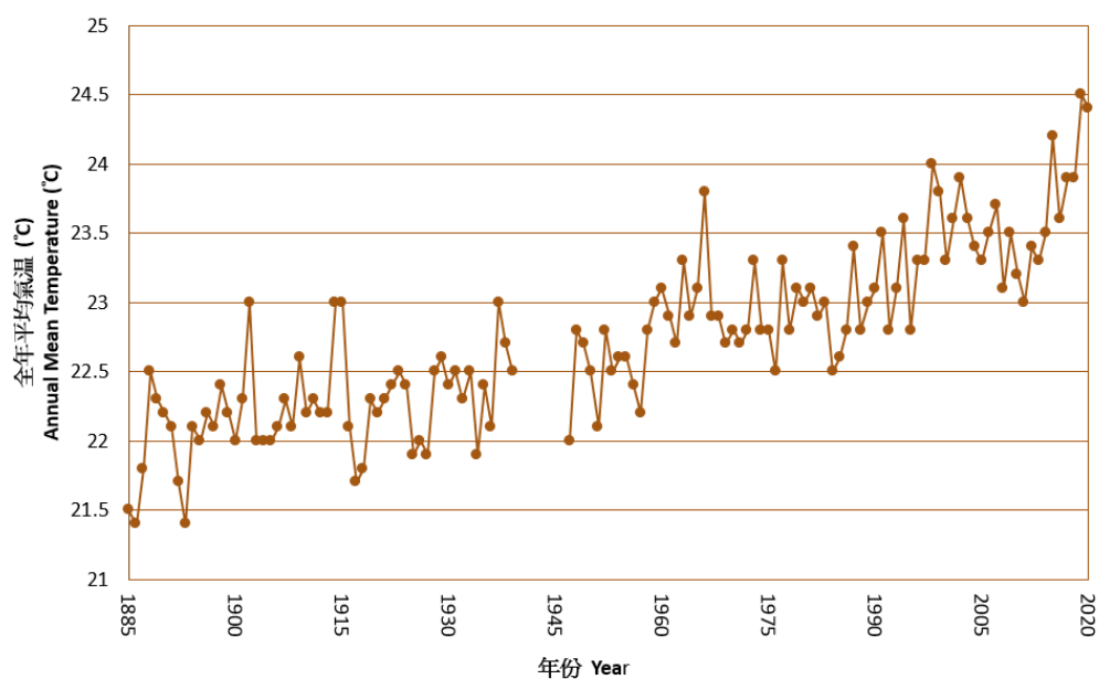
圖表五 香港全年平均氣溫的長期時間序列(一八八五至二〇二〇年)
