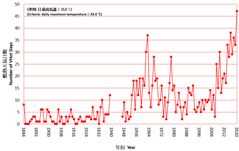
圖表三 香港全年酷熱天氣日數的長期時間序列（一八八四至二〇二〇年）
