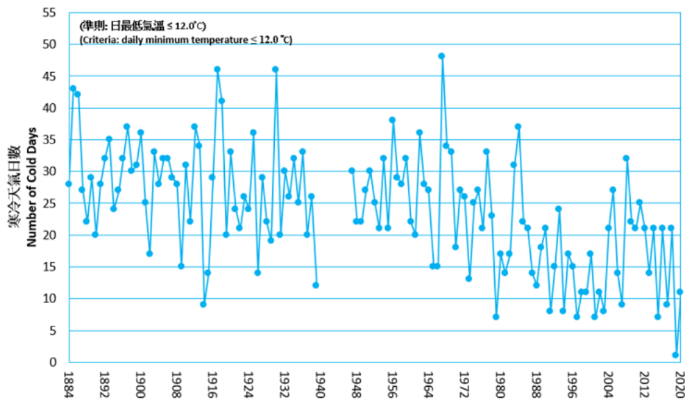
圖表四 香港全年寒冷天氣日數的長期時間序列（一八八四至二〇二〇年）
