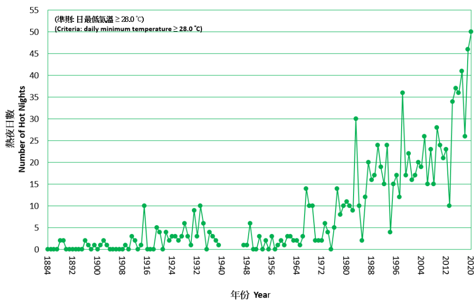
圖表二 香港全年熱夜數目的長期時間序列（一八八四至二〇二〇年）
