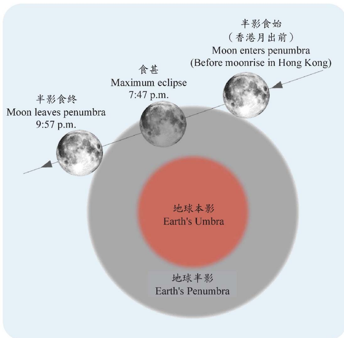
三月二十三日半影月食時月球的路徑
