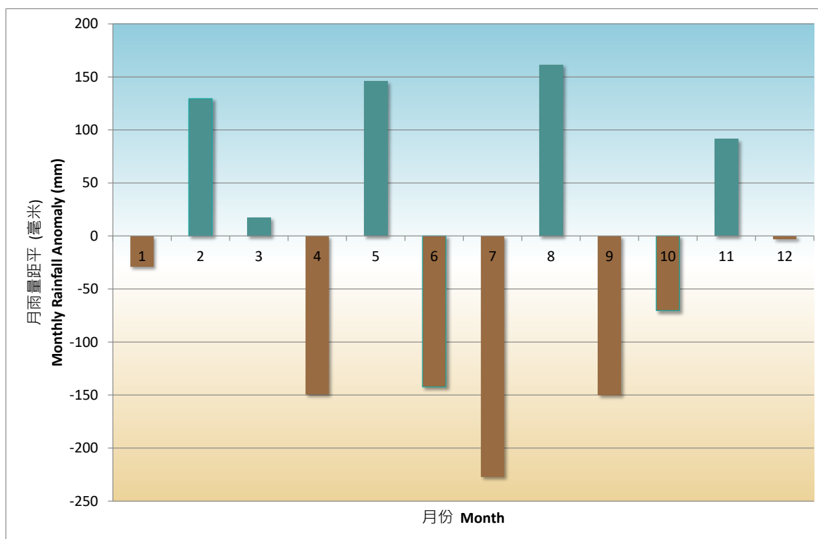
圖六 二〇二二年香港月雨量距平（與一九九一至二〇二〇年正常值相比）
