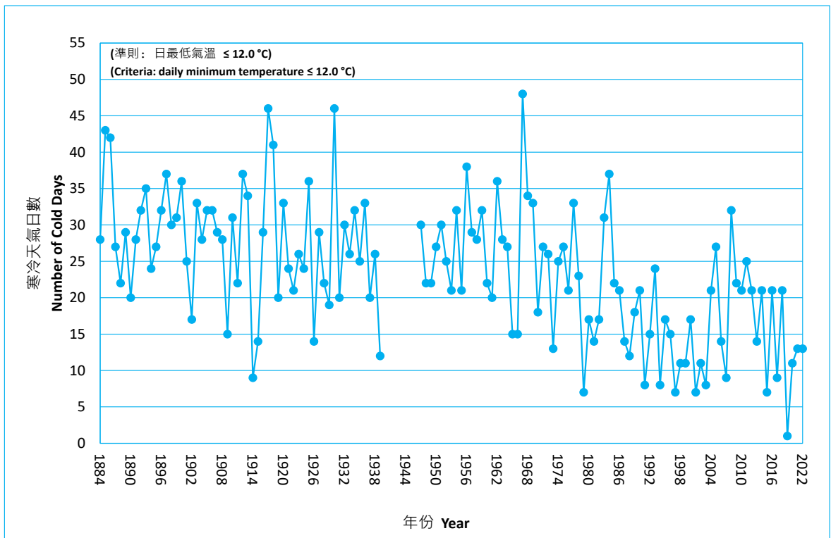
圖四 香港全年寒冷天氣日數的長期時間序列（一八八四至二〇二二年）
