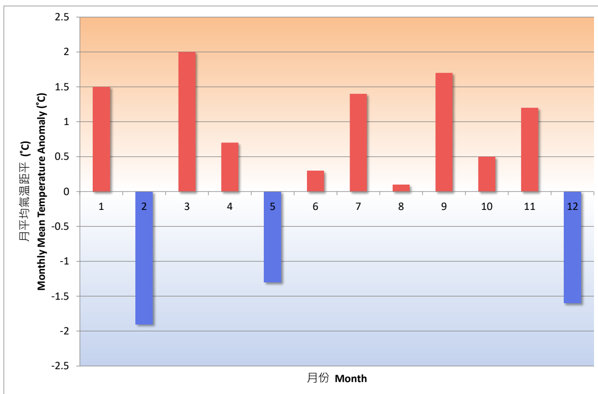
圖一 二〇二二年香港月平均氣溫距平（與一九九一至二〇二〇年正常值相比）
