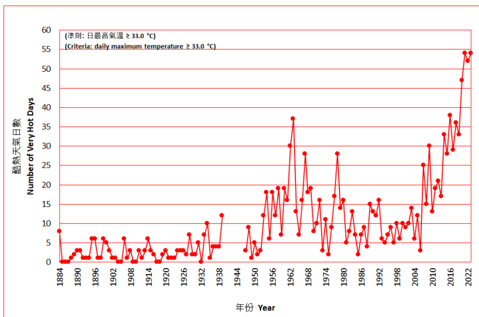
圖三 香港全年酷熱天氣日數的長期時間序列（一八八四年至二〇二三年）
