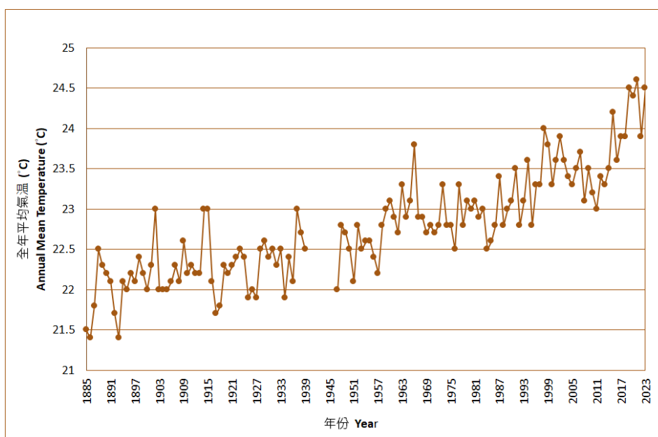
圖六 香港全年平均氣溫的長期時間序列（一八八五年至二〇二三年）
