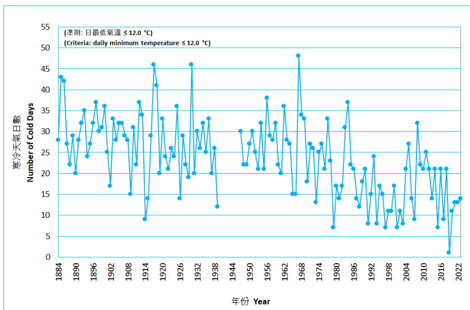
圖五 香港全年寒冷天氣日數的長期時間序列（一八八四年至二〇二三年）
