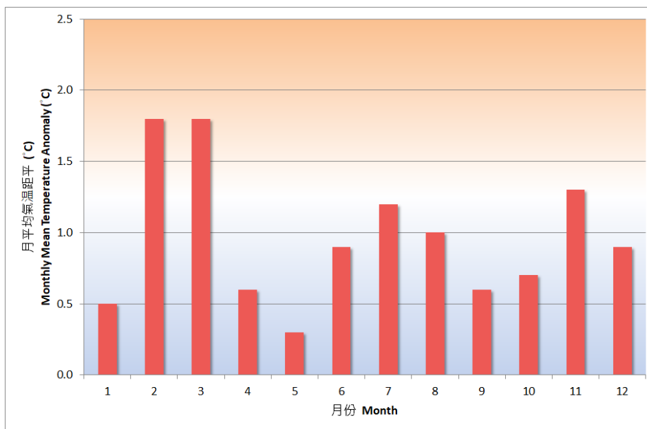
圖一 二〇二三年香港月平均氣溫距平（與一九九一年至二〇二〇年正常值相比）
