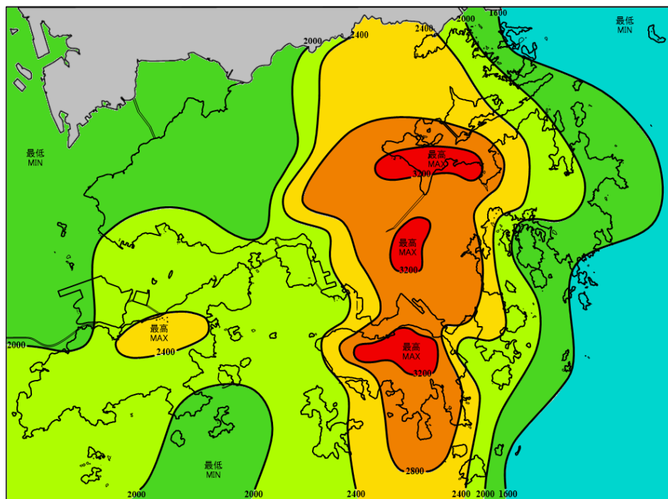
圖八 二〇二三年香港年雨量分佈（毫米）
