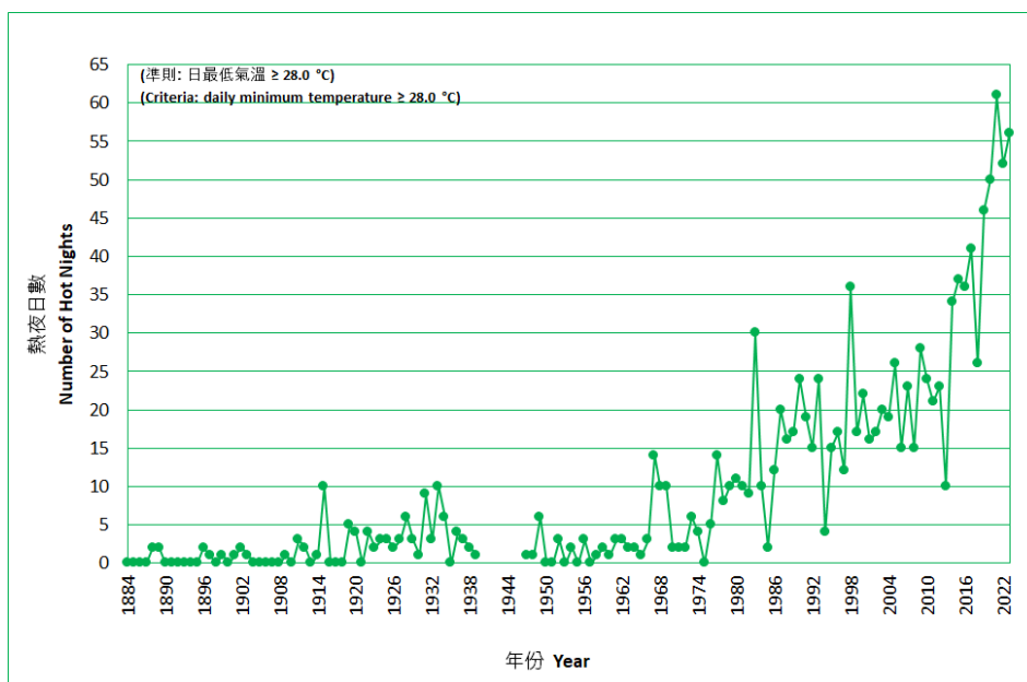
圖二 香港全年熱夜數目的長期時間序列（一八八四年至二〇二三年）
