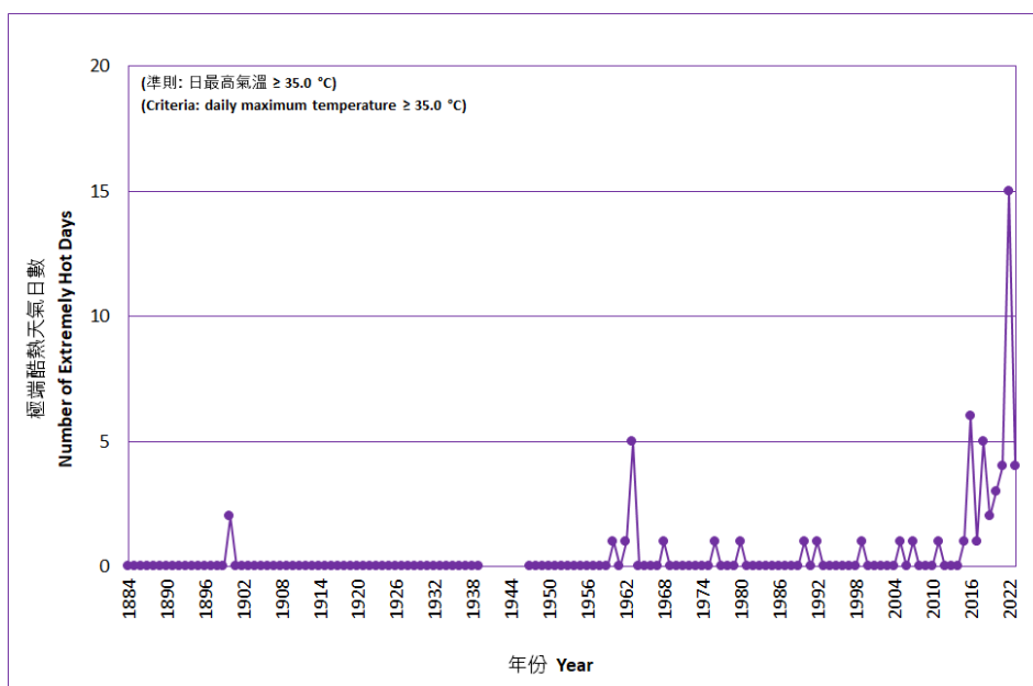
圖四 香港全年極端酷熱天氣日數的長期時間序列（一八八四年至二〇二三年）
