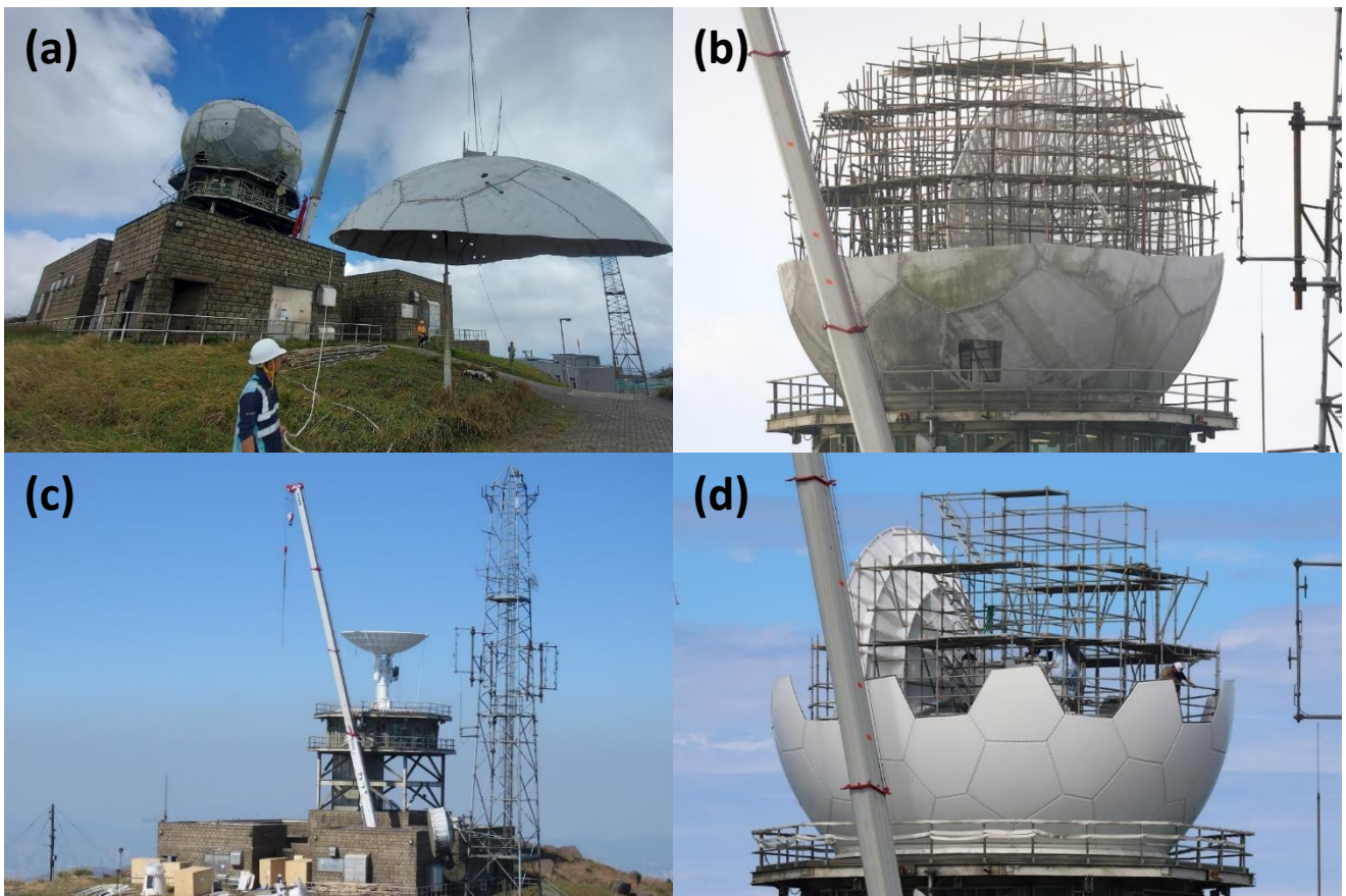
圖三 (a)拆卸舊大帽山天氣雷達天線罩，(b)工人搭建棚架用以拆卸舊的雷達天線，(c)安裝新雷達的天線及基座，(d)構建中的新雷達天線罩。
