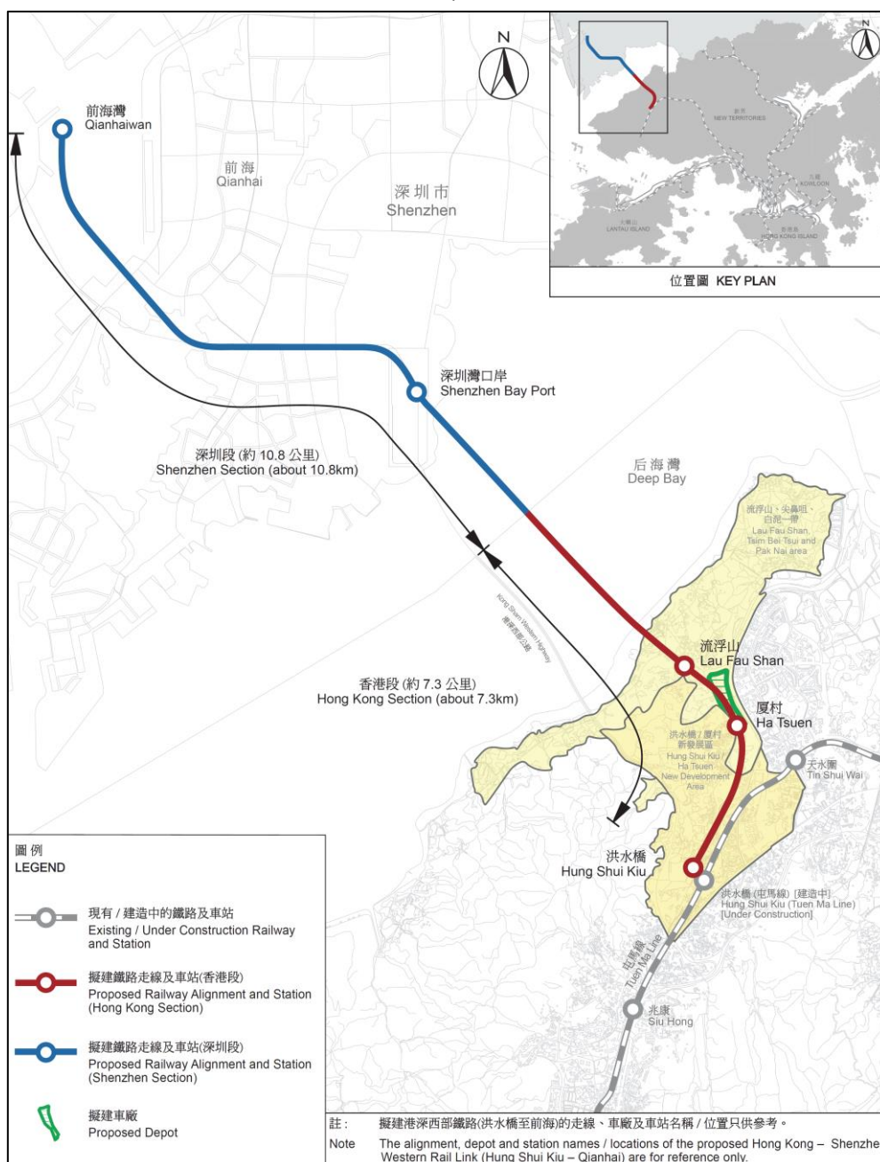
港深西部鐵路 ( 洪水橋至前海 ) 初步走線
